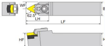
寸法 Dimension(mm)
