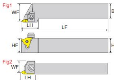
寸法 Dimension(mm)
