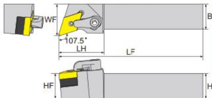
寸法 Dimension(mm)
