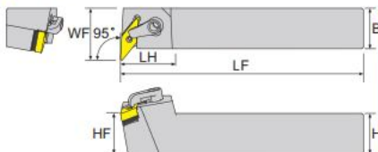
寸法 Dimension(mm)
