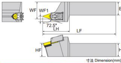
寸法 Dimension(mm)
