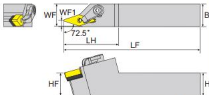
寸法 Dimension(mm)
