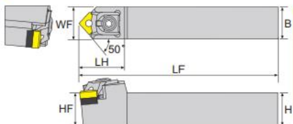
寸法 Dimension(mm)
